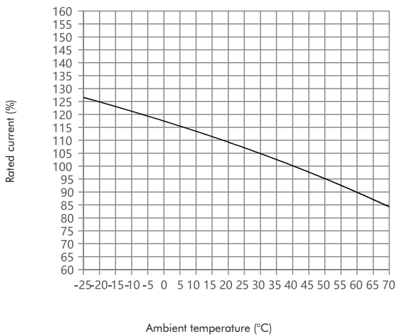
NXMLE-125 16A~25A
