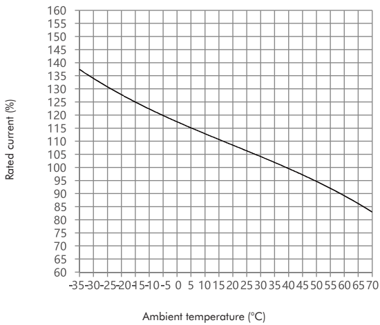
NXMLE-160(W125) 25A-63A
