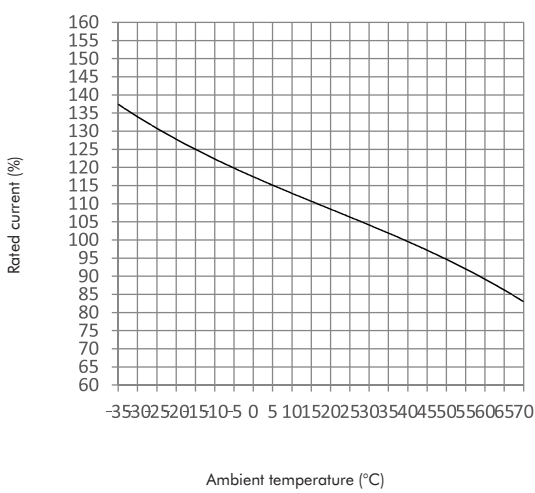
NXMLE-160(W125) 16A-20A
